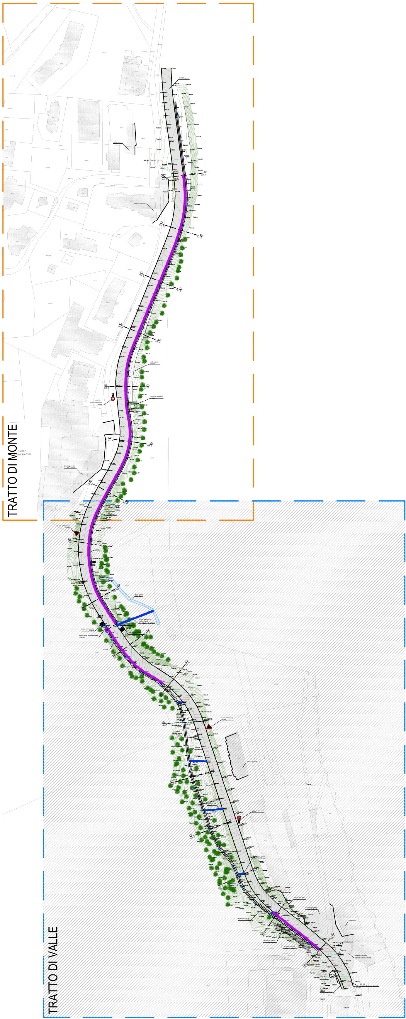
PLANIMETRIA GENERALE - scala 1:2.000
